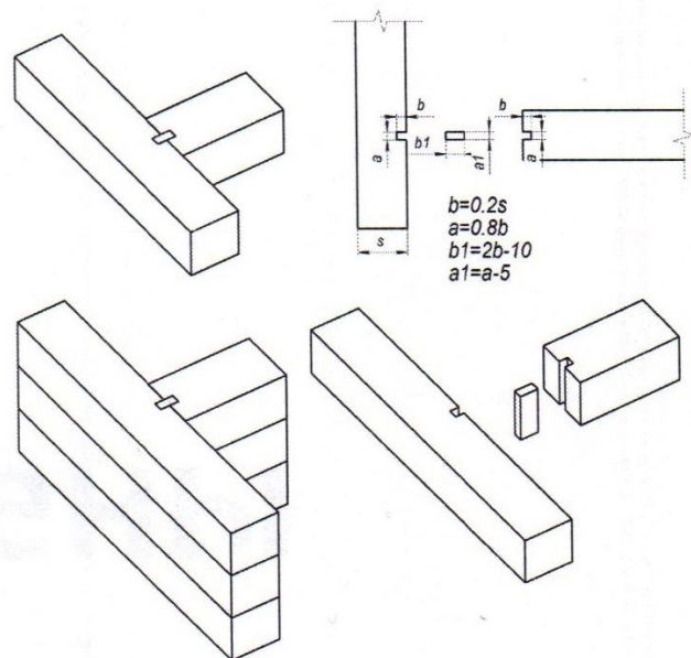
Вставной шип с прямой подрезкой
